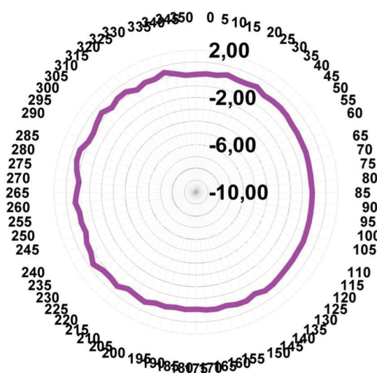
Freq. 900 MHz H-plane (dBi) V-pol
