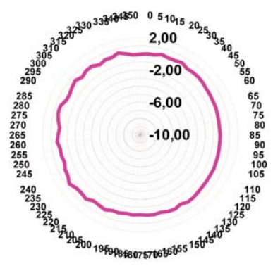
Freq. 900 MHz H-plane (dBi) V-pol
