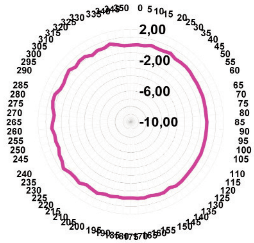
Freq. 900 MHz H-plane (dBi) V-pol
